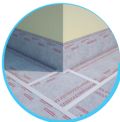
ANGOLO ESTERNO 270°
